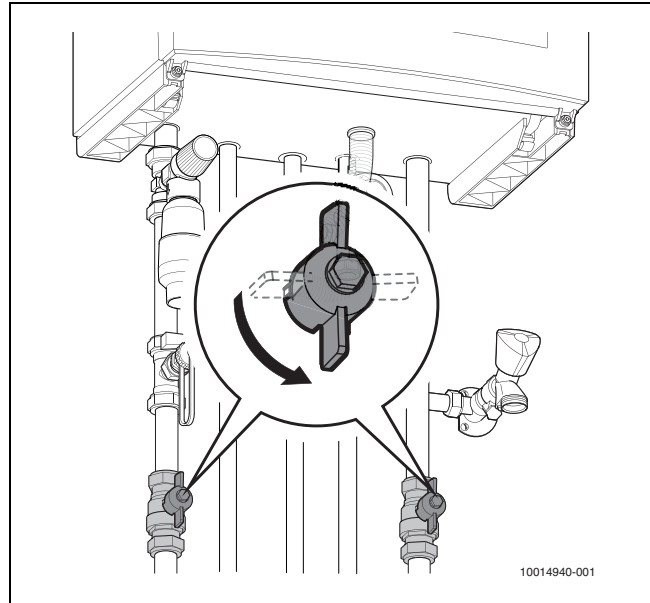
Afb. 4 Serviceafsluiters
