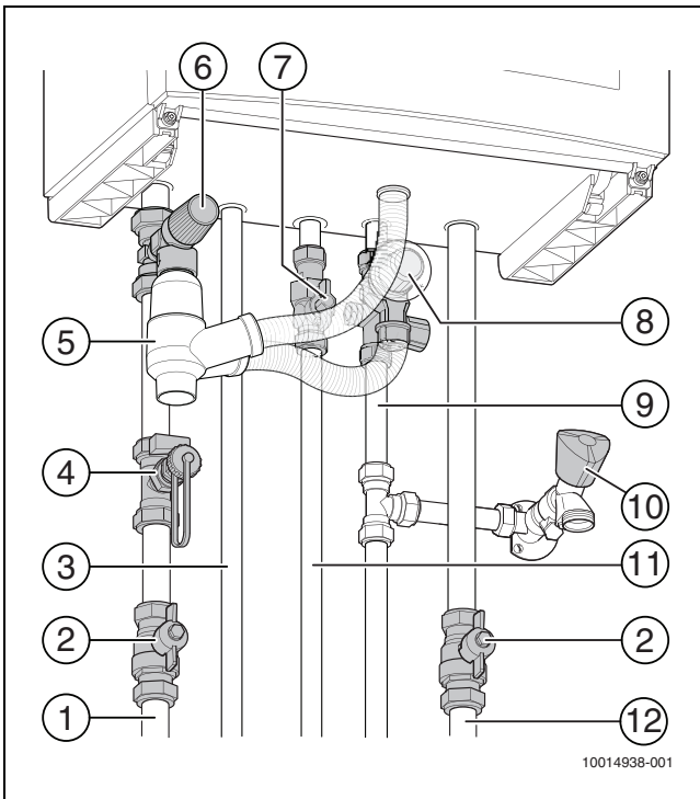
Afb. 2 Overzicht aansluitingen
